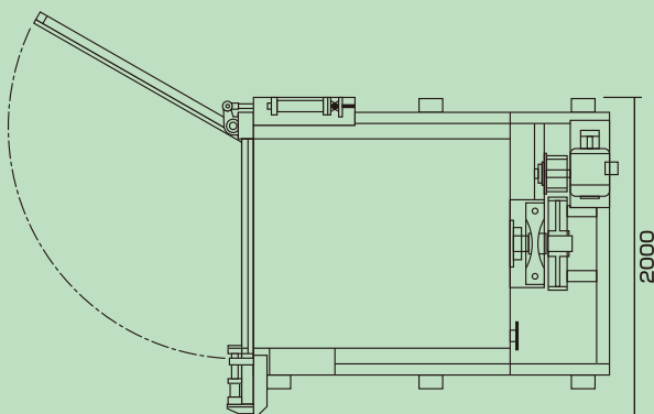
ドラムクリーニングマシン(ODR-140型)
