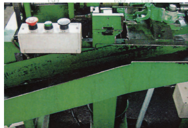
処理済みクランプをストック用の袋へ流すシュート
